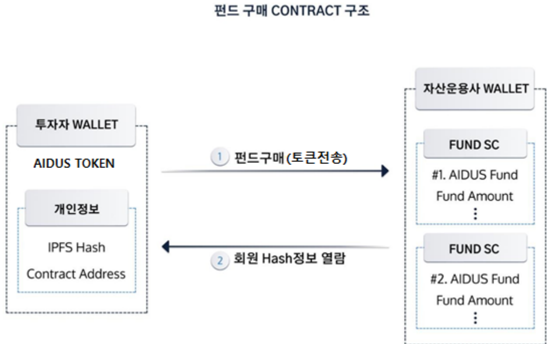
[ 그림 35 ] 펀드 구매 CONTRACT 구조도
