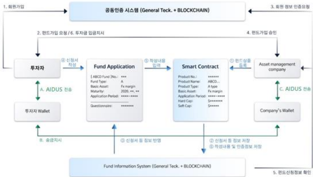
[ 그림 31 ] ADFP 기반 탈중양화 펀드마켓 기본 기능 구조
